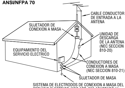
EJEMPLO DE CONEXION A MASA DE LA ANTENA DE ACUERDO CON EL CODIGO ELECTRICO NACIONAL, ANSI/NFPA 70
